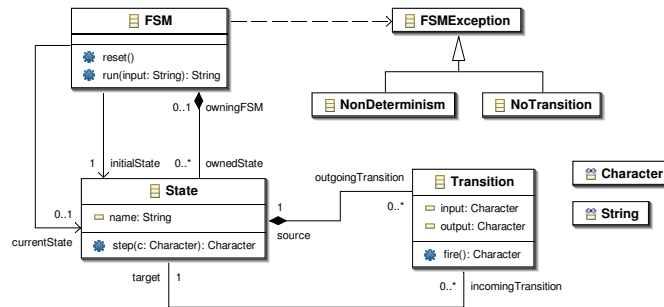
Fig. 11. Simple FSM metamodel
